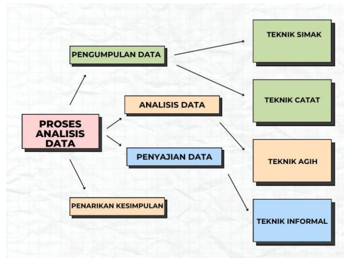
Gambar 1. Pendekatan Metodologis.
